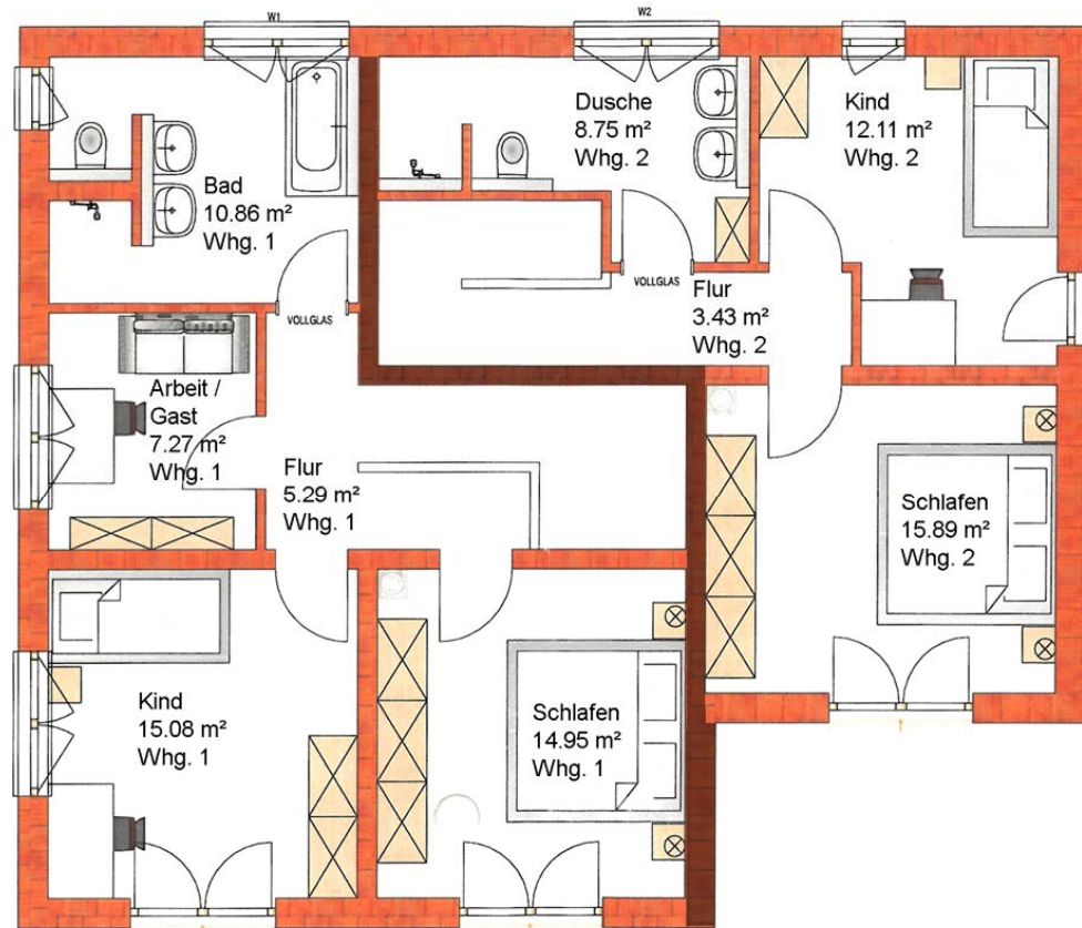
Obergeschoss
